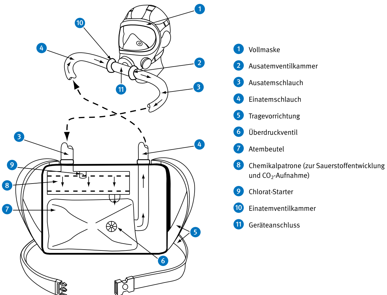
Abb. 42 Chemikalsauerstoff(KO 2 )schutzgerät
